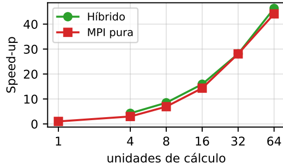
(a) Escalabilidade forte
