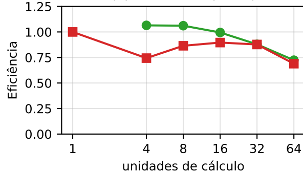
(c) Eficiência (forte)
