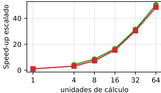
(b) Escalabilidade fraca (speed-up)
