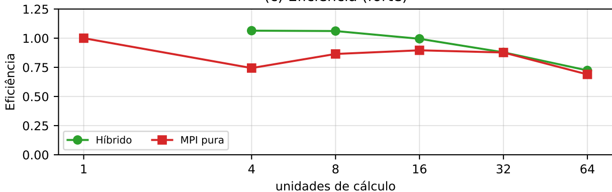
(c) Eficiência (forte)
