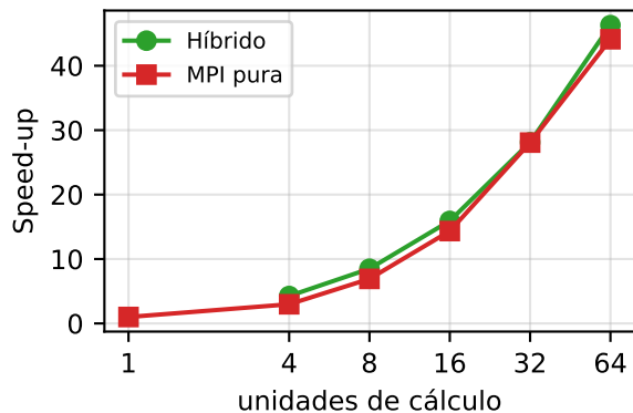
(a) Escalabilidade forte
