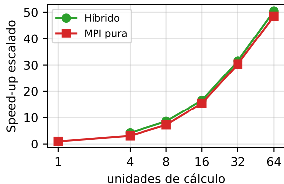
(b) Escalabilidade fraca (speed-up)
