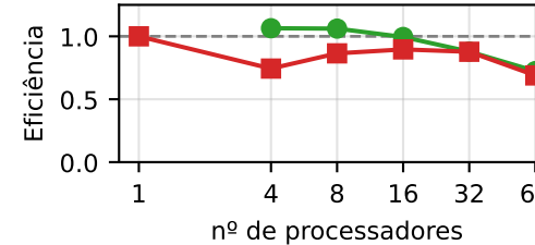
(c) Eficiência (forte)
