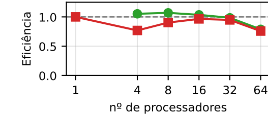
(d) Eficiência (fraca)
