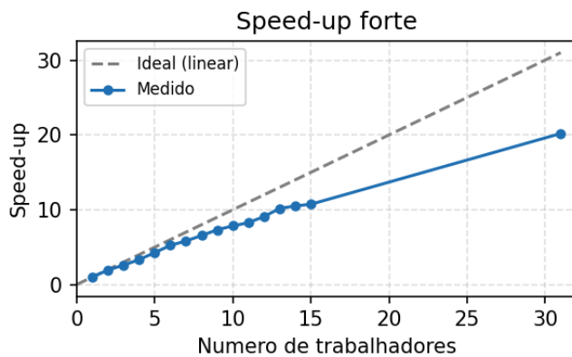
Fig. 1 — Speed-up (escala forte)
