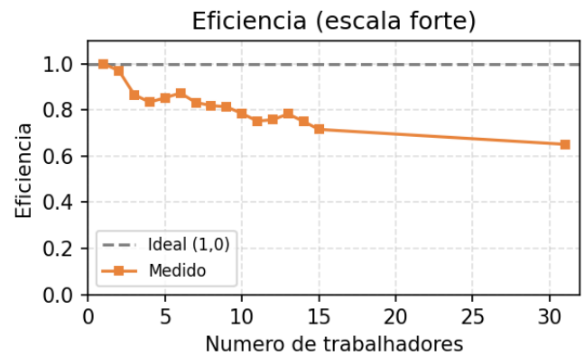
Fig. 2 — Eficiência (escala forte)
