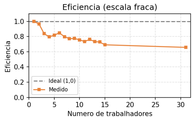
Fig. 4 — Eficiência (escala fraca)
