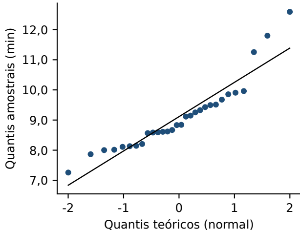
Gráfico Q-Q normal
