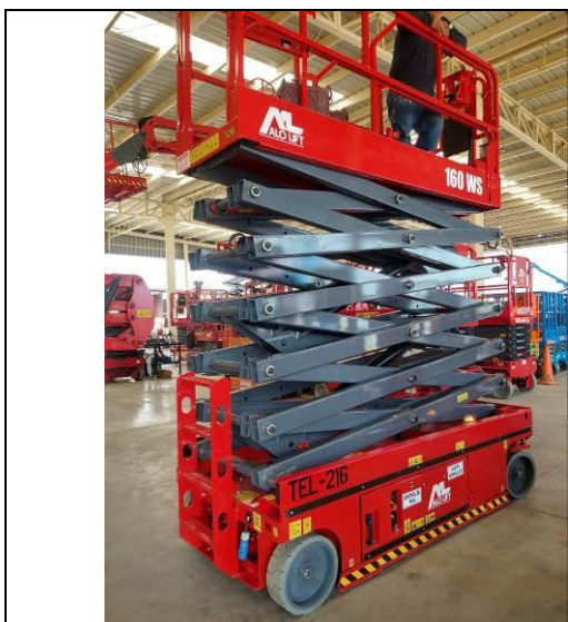
Foto N° 5 PRUEBA DE ELEVACION CON CARGA
