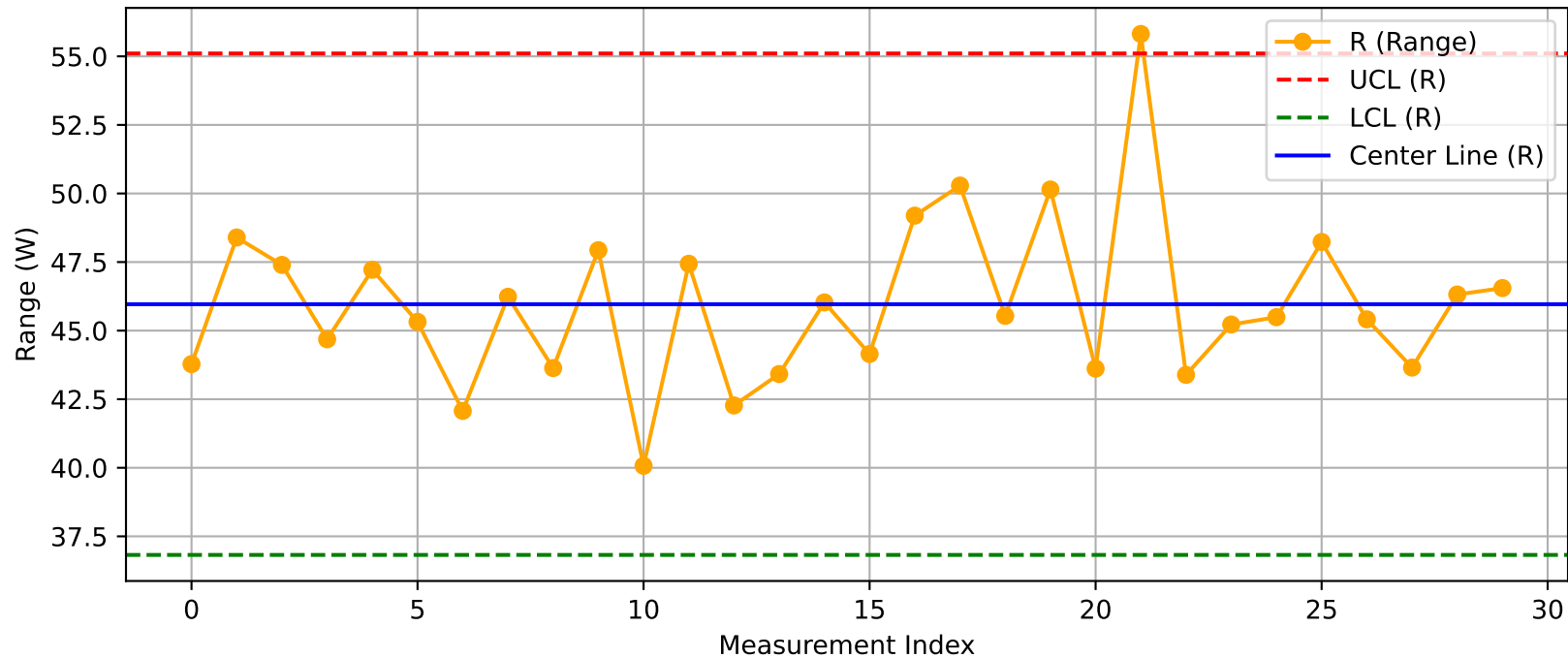
DUT - R Chart (T40_Test200@Test.xlsx)
