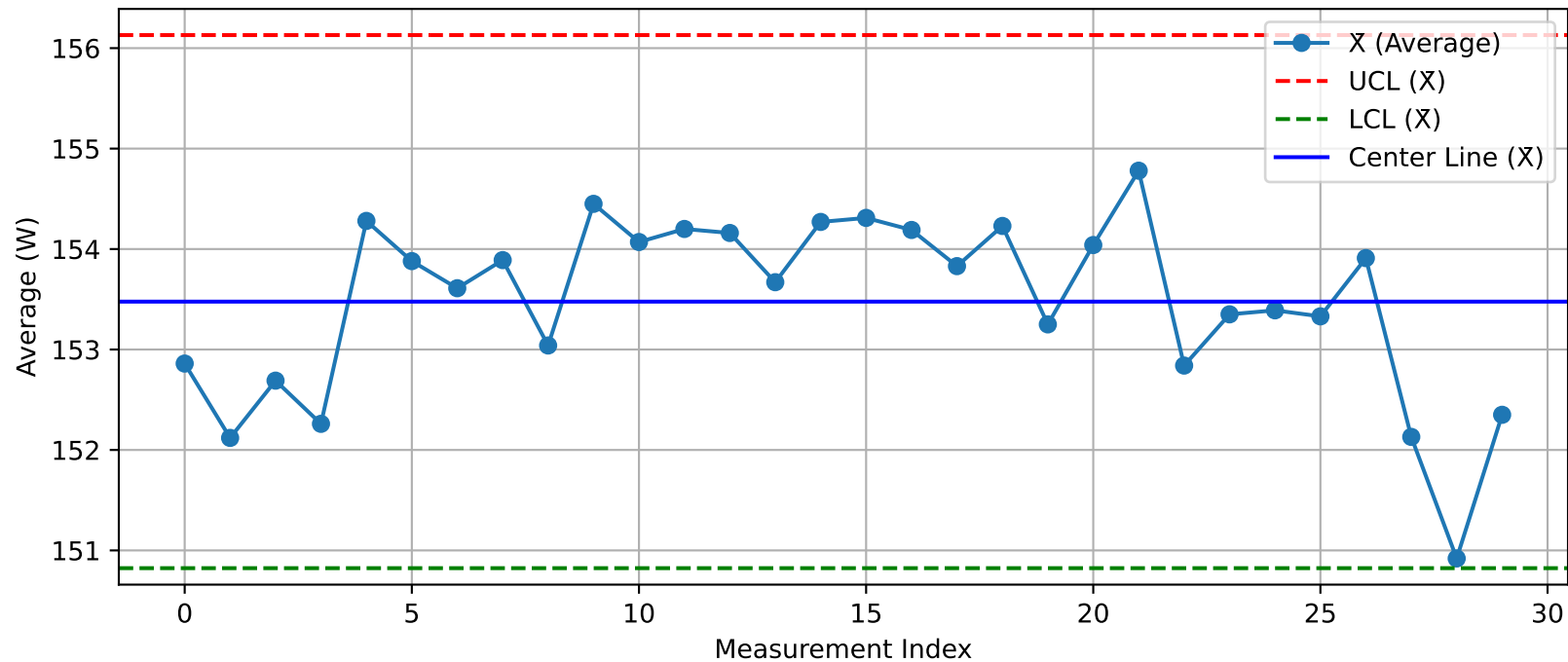
DUT - \bar{X} Chart (T20@Test2.xlsx)
