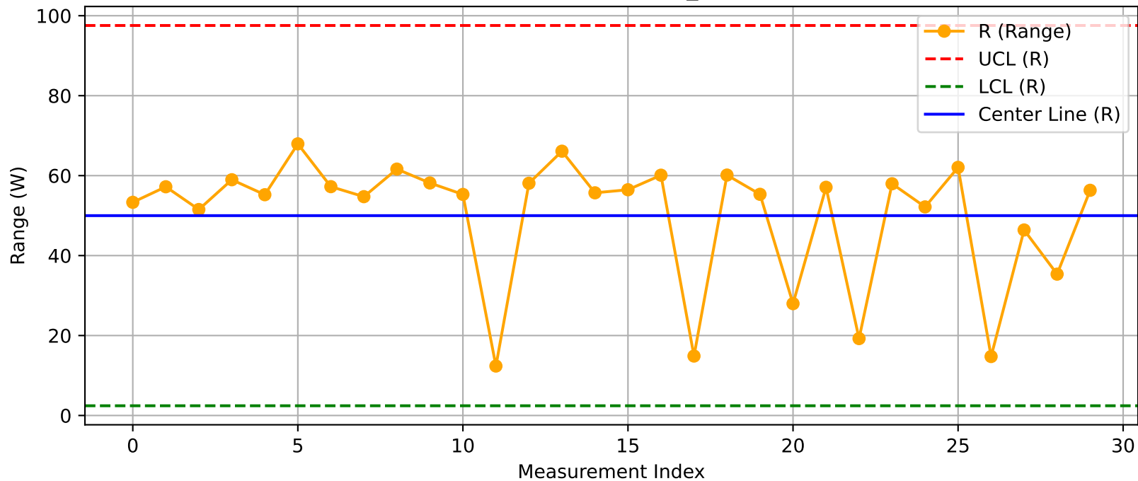
DUT - R Chart (T40@Test1_Nuitka.xlsx)
