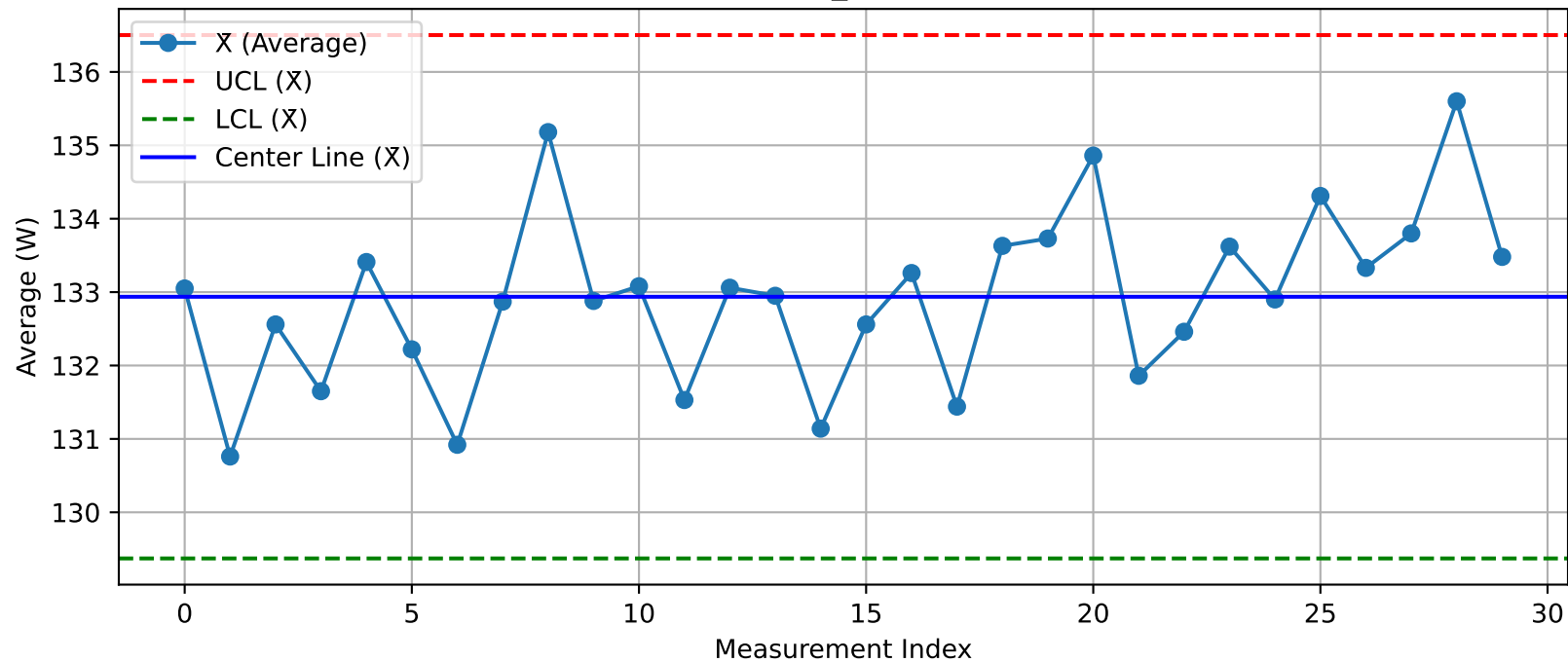
DUT - \bar{X} Chart (T04_Test100@Test.xlsx)
