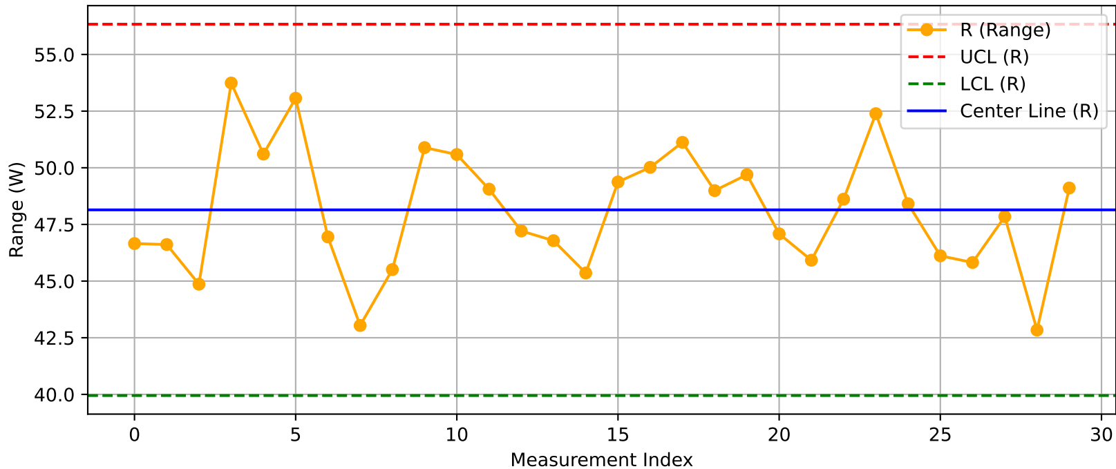
DUT - R Chart (T40_Test100@Test.xlsx)
