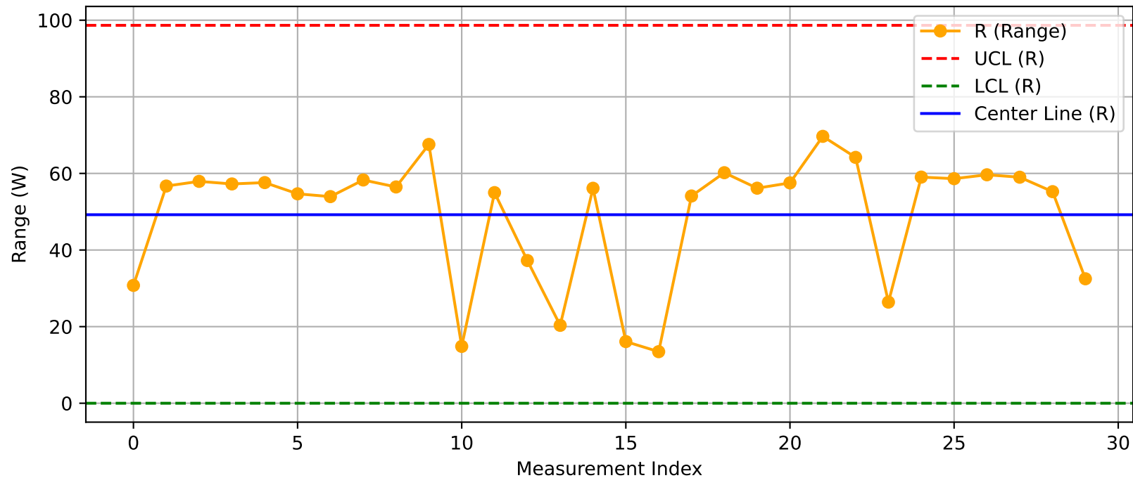
DUT - R Chart (T40@Test1.xlsx)
