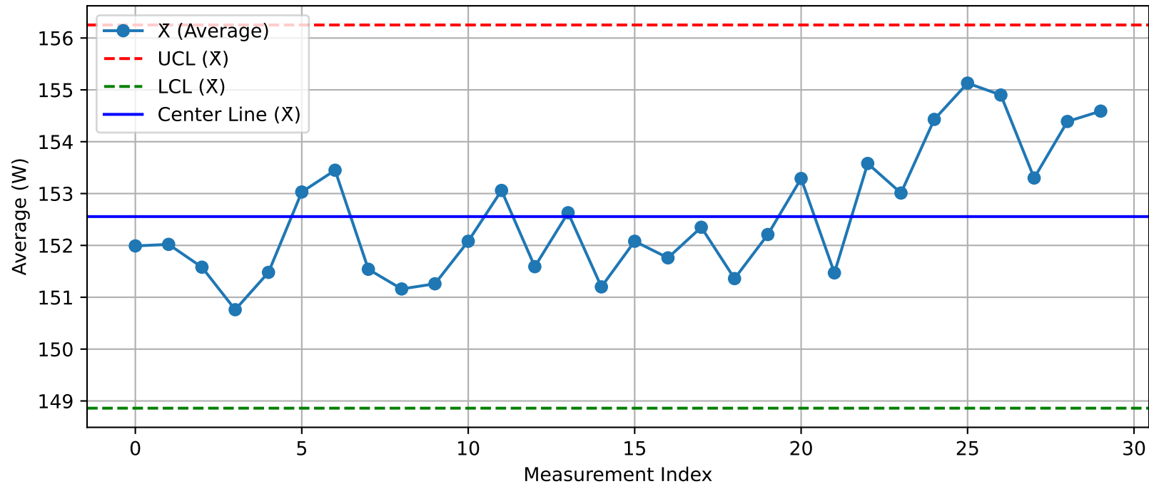
DUT - \bar{X} Chart (T40@Test1_Nuitka.xlsx)
