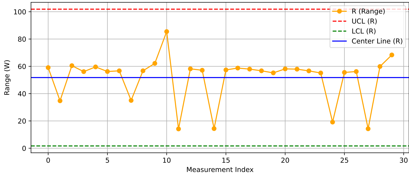
DUT - R Chart (T40@Test2.xlsx)
