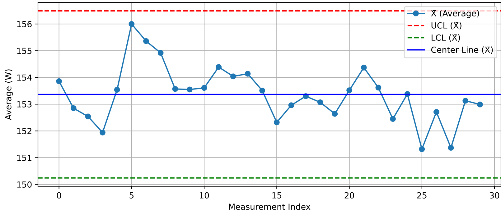
DUT - \bar{X} Chart (T40@Test2_Nuitka.xlsx)
