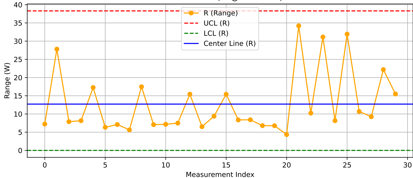
DUT - R Chart (T9@Test2.xlsx)
