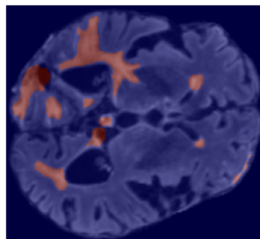
3pi3 61
