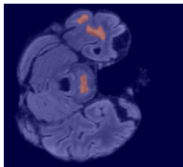
3pi3 35
