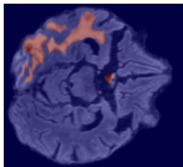
3pi3 45
