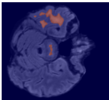
3pi3 38
