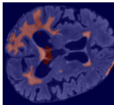
3pi3 71
