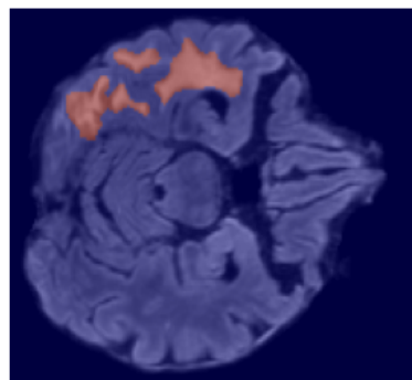
3pi3 42
