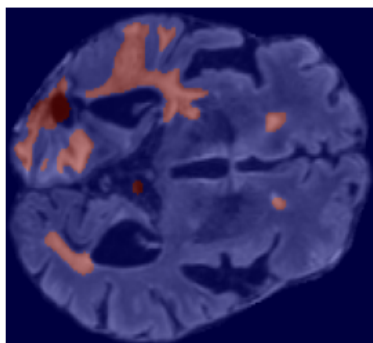
3pi3 58
