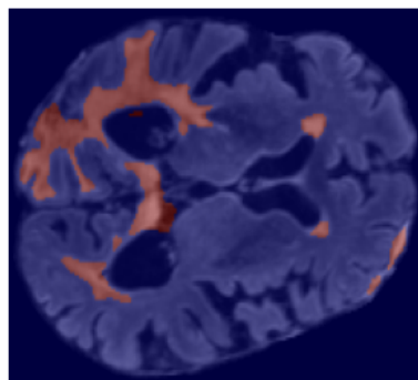
3pi3 65
