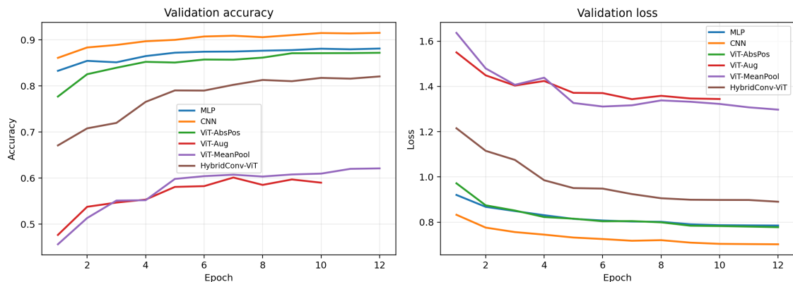
图 12: 六组模型最新一次正式训练的验证准确率与验证损失
