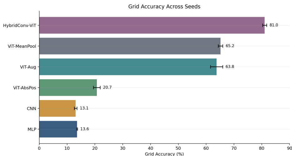
图 9: 五个随机种子下六组模型的 49 点 Grid Accuracy 均值与标准差
