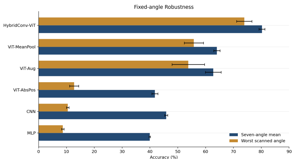
图 11: 五个随机种子下固定角度扫描的七角度平均值与最差角度
