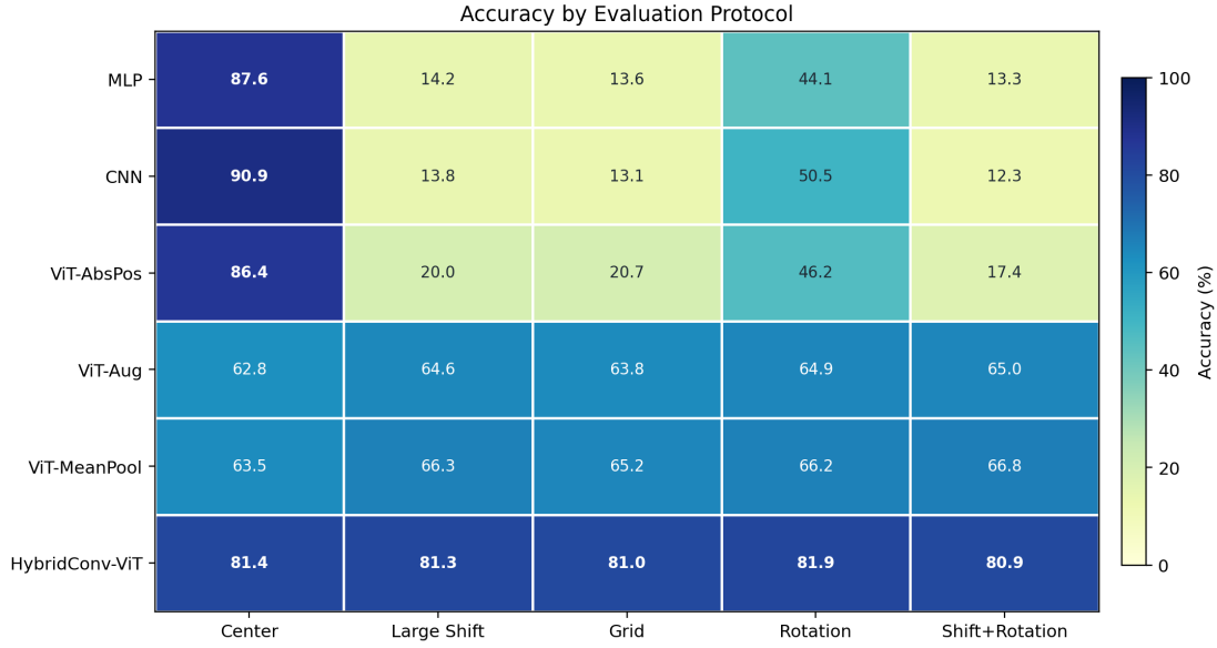
图 8: 五个随机种子汇总后的多协议 Accuracy。单元格数字为均值百分比，标准差见表 4
