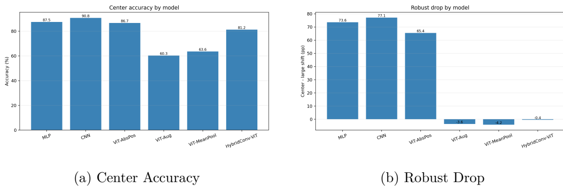
图 8: 中心准确率与大平移鲁棒性
