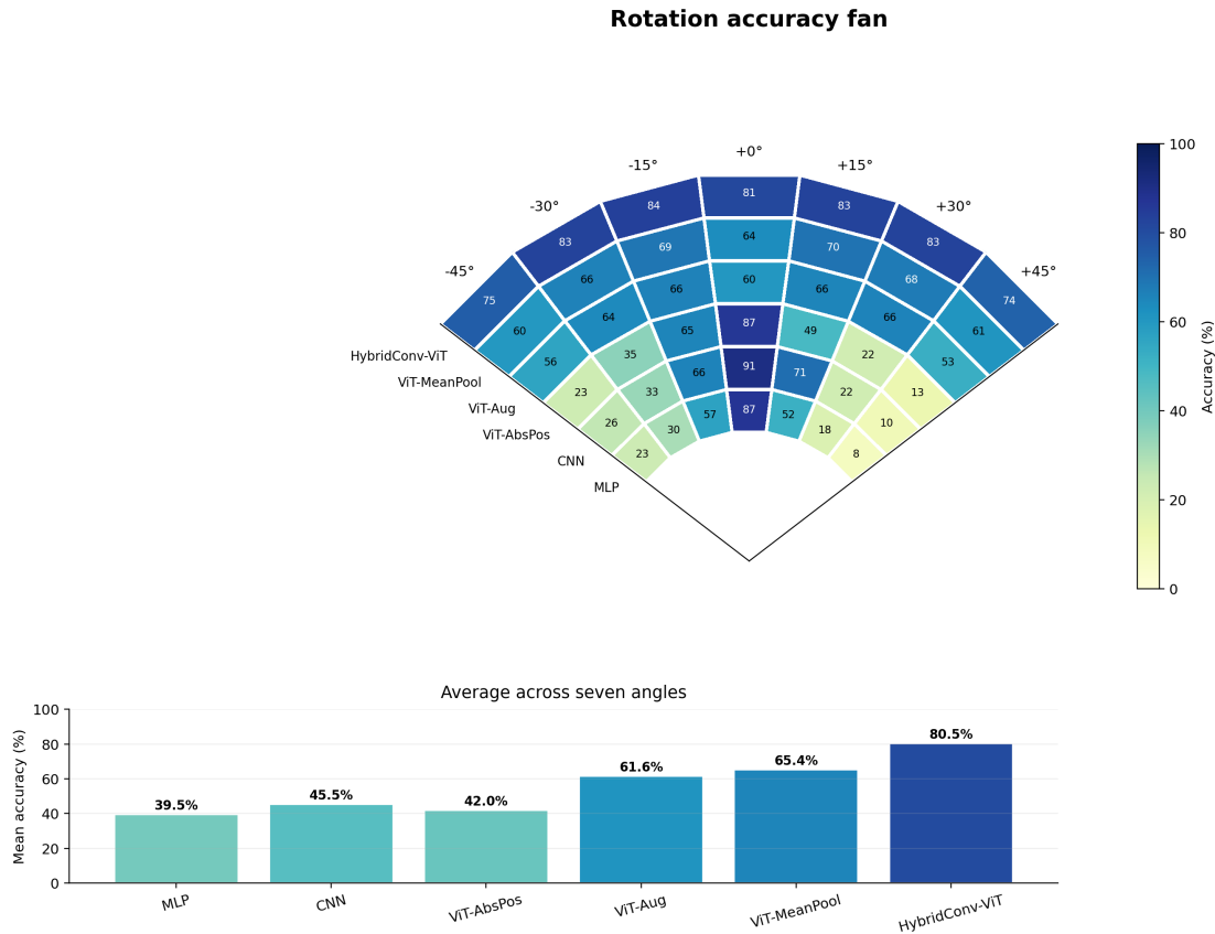
图 13: 固定角度扇形热力图与七角度平均准确率：扇形由左至右对应 -45^{\circ} 到 45^{\circ} ，颜色和数字共同表示 Accuracy
