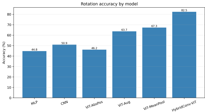
图 10: 六组模型在连续随机旋转协议下的 Rotation Accuracy
