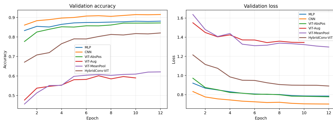
图 11: 六组模型最新一次正式训练的验证准确率与验证损失
