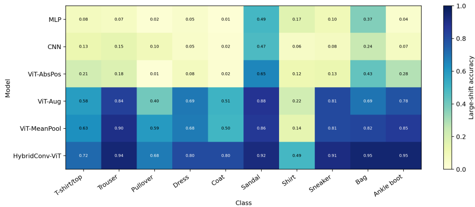
图 14: Large Shift 条件下的逐类准确率
