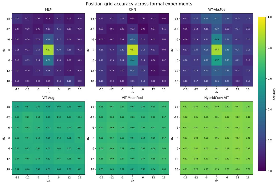
图 12: 六组模型的 7 \times 7 位置网格准确率：横轴和纵轴分别为 dx 、 dy ，每个单元均来自完整测试集
