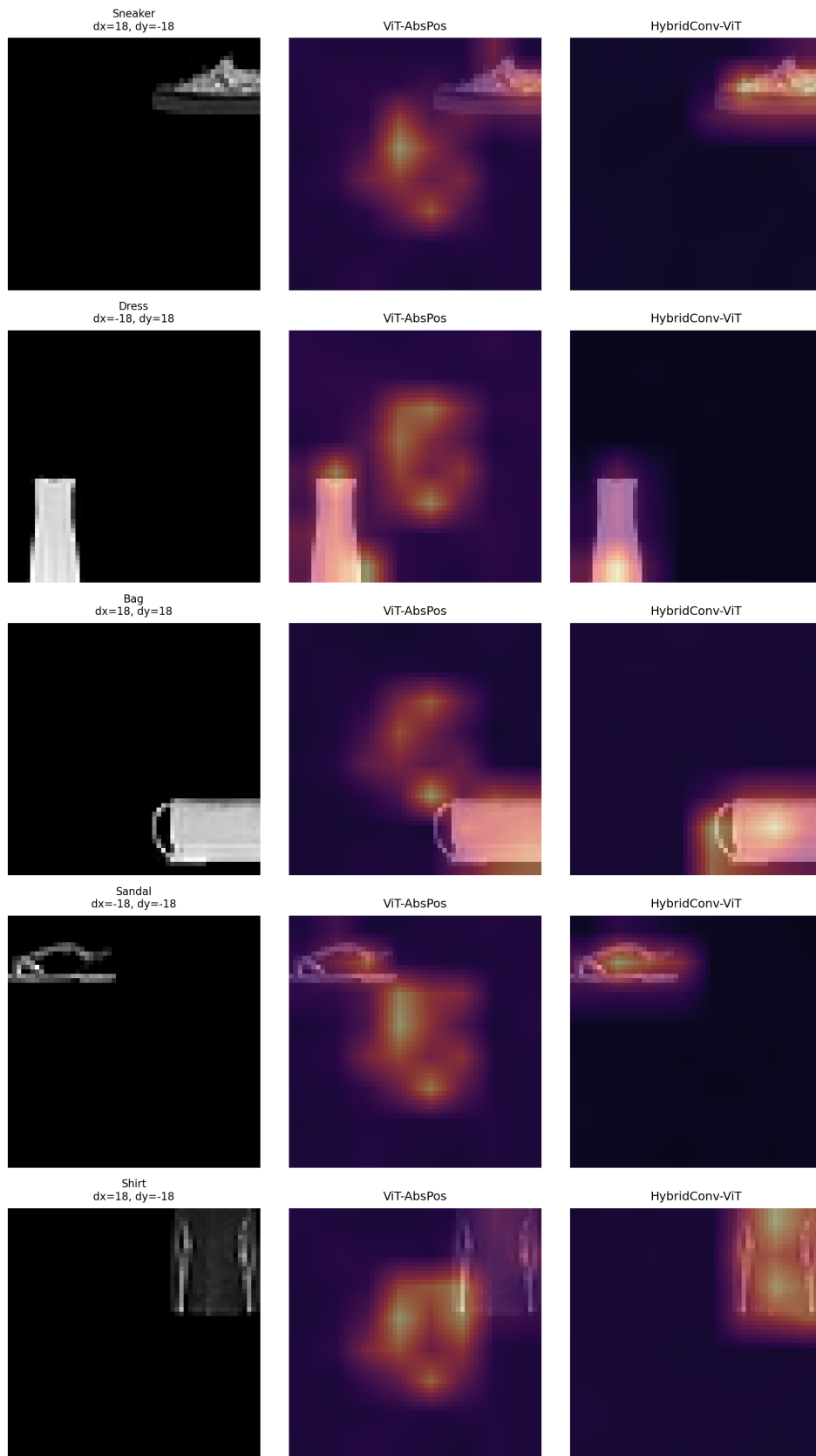
图 19: 随机种子 42 中五个边缘位置样本的 Attention Rollout 对照 (二)
