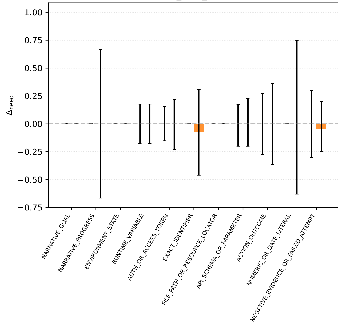
general_task_agnostic
