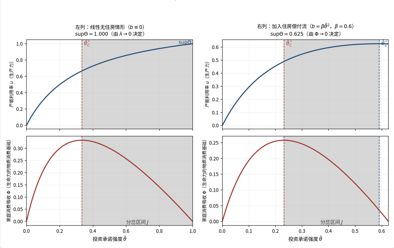
图1 边际分岔区间： \varepsilon_u > 0 > \varepsilon_\Phi ( c = 0.75 , \mu = 1 , \iota = 0 , \bar{u} = 1 ；横轴止于经济可行域上界；示例，非估计)
