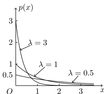
图 2.3: 参数为 \lambda 的指数分布密度函数
