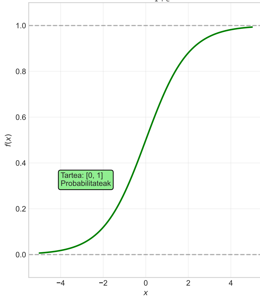
Sigmoid: \frac{1}{1 + e^{-x}}
