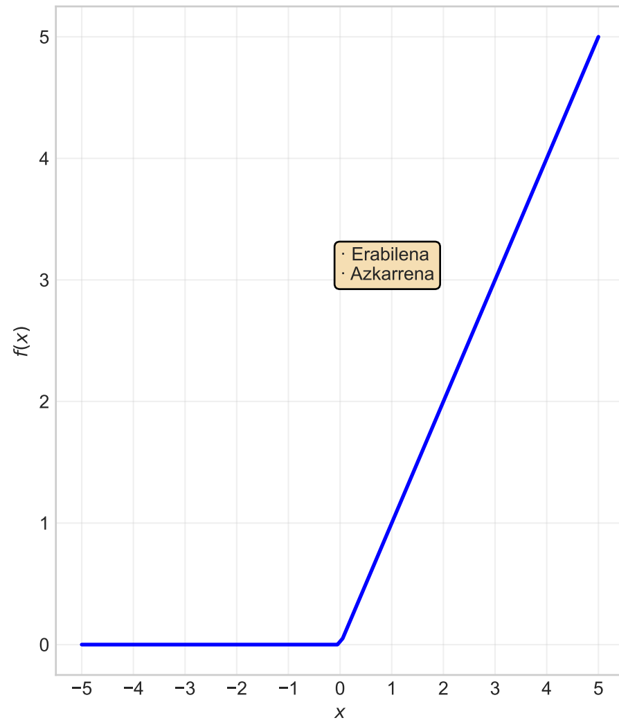
ReLU: \max(0, x)
