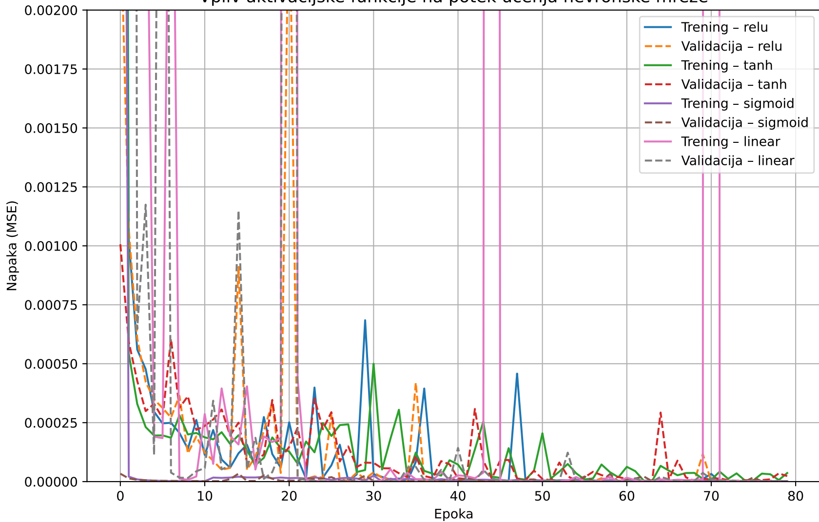
Vpliv aktivacijske funkcije na potek učenja nevronske mreže
