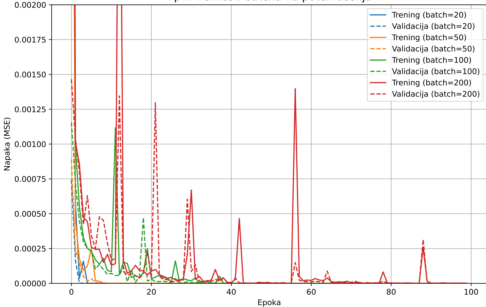
Vpliv velikosti batcha na potek učenja
