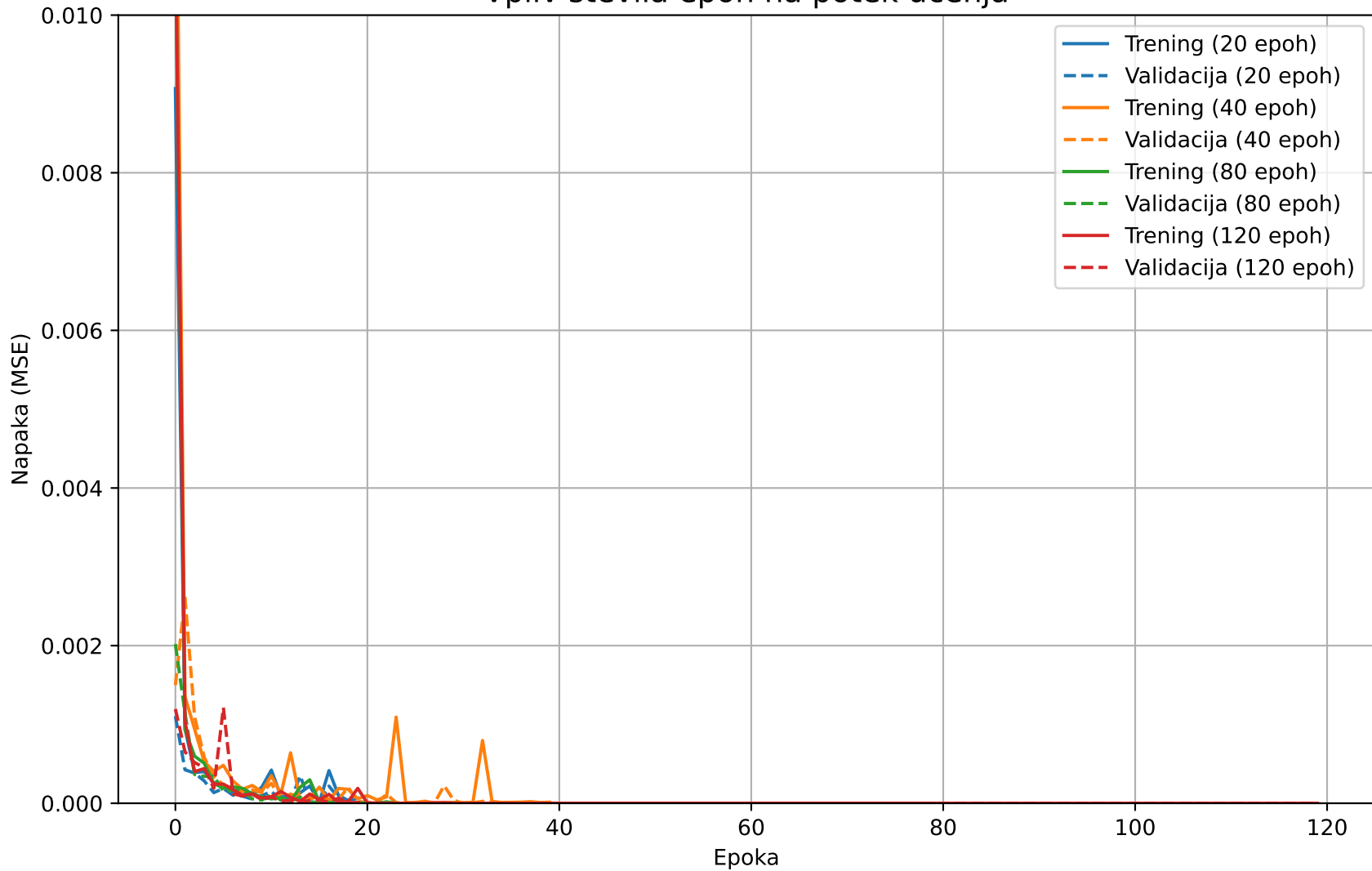
Vpliv števila epoh na potek učenja
