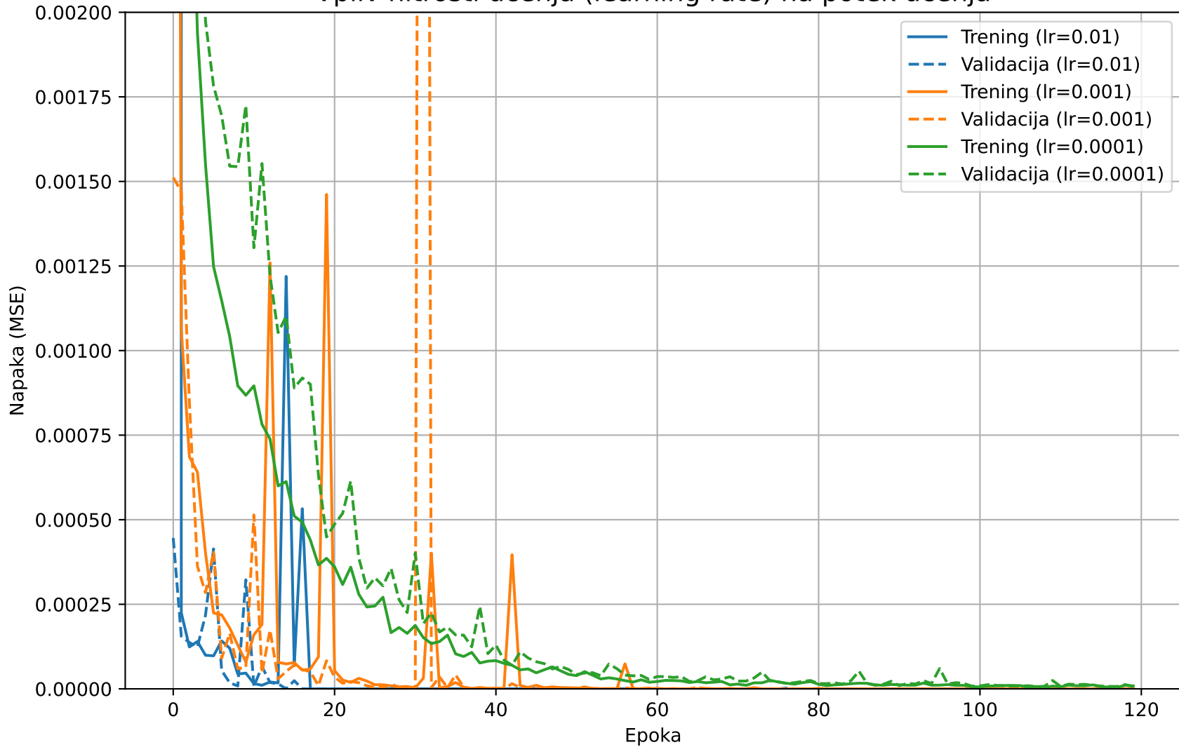
Vpliv hitrosti učenja (learning rate) na potek učenja
