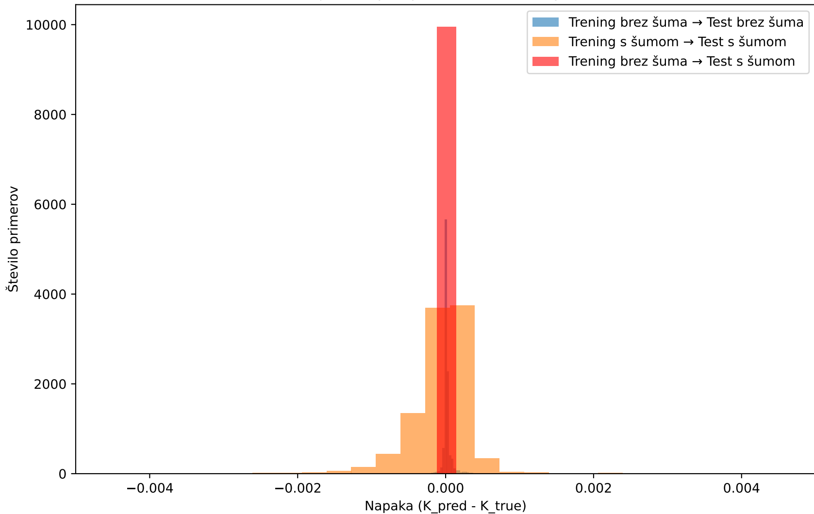
Primerjava napak pri različnih učnih podatkih
