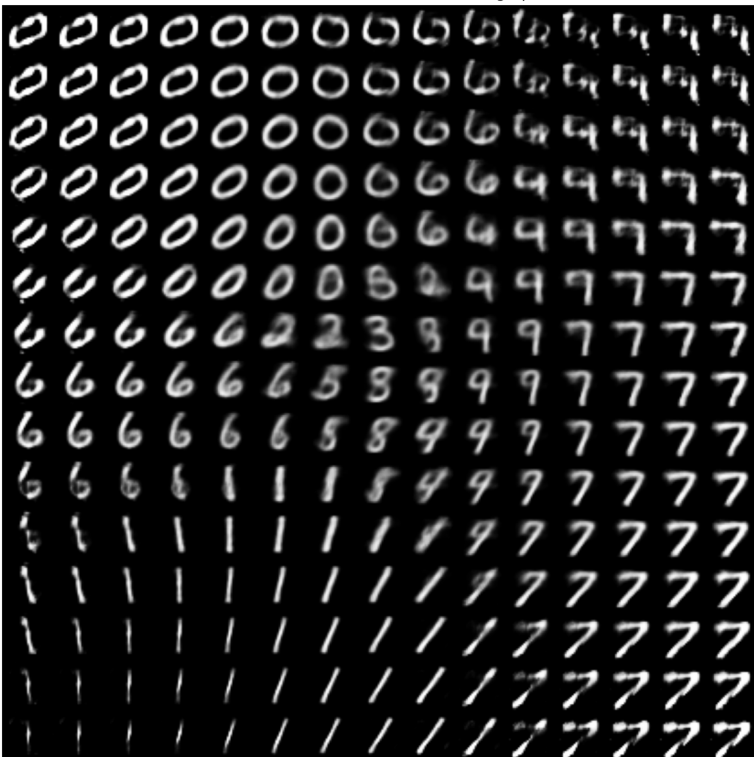
Generirane številke iz 2D mreže latentnega prostora
