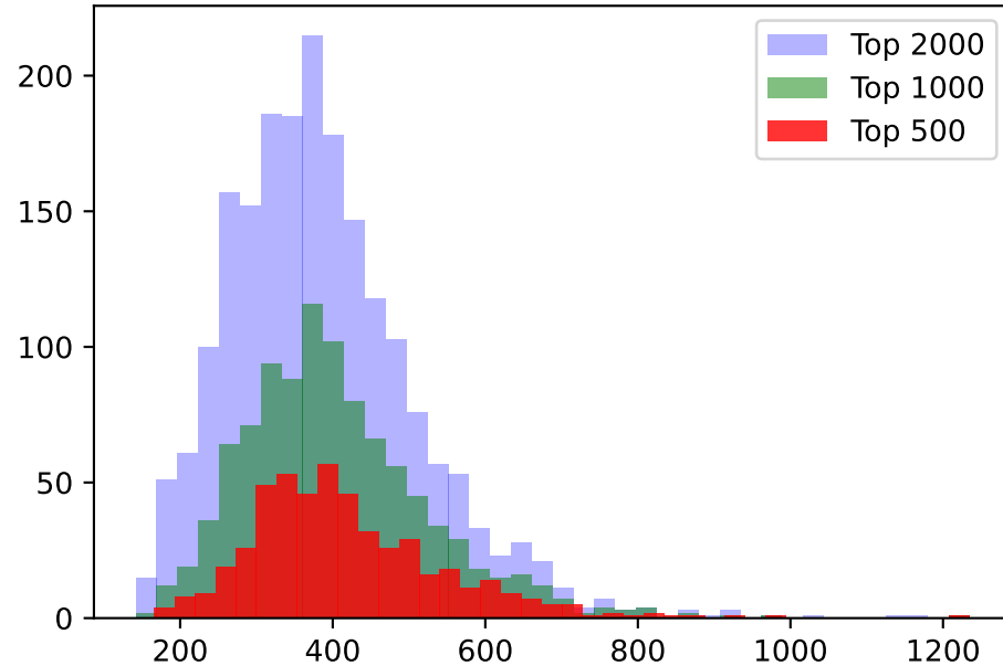
Masa 2. curka ( m_{j2} )
