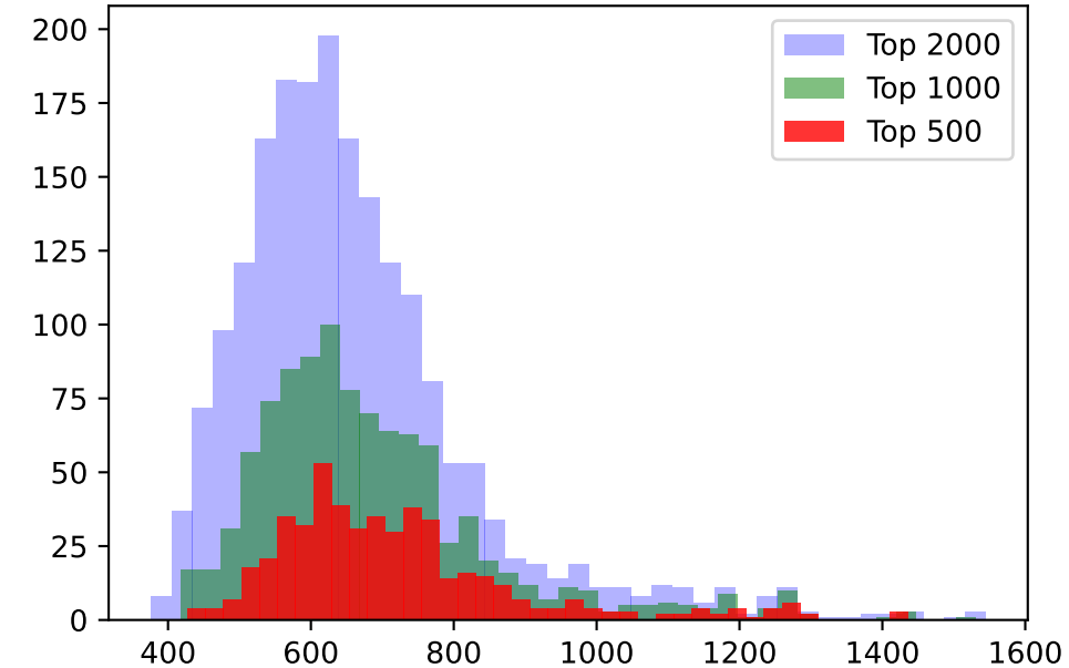
Masa 1. curka ( m_{j1} )
