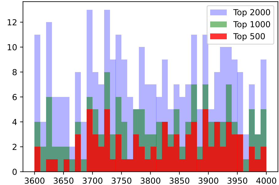
Invariantna masa ( m_{inv} )
