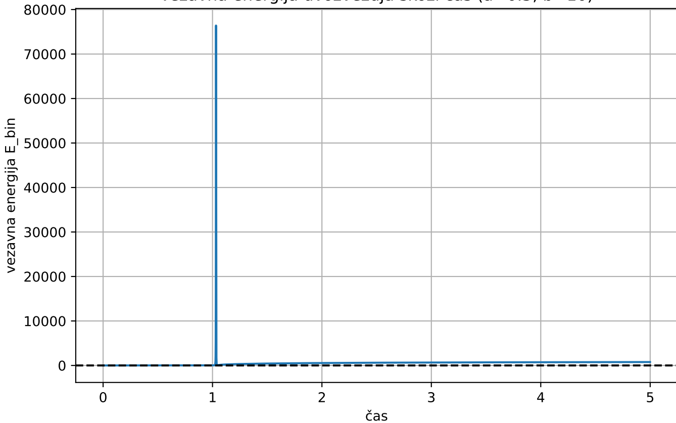
Vezavna energija dvozvezdja skozi čas ( a=0.5 , b=10 )
