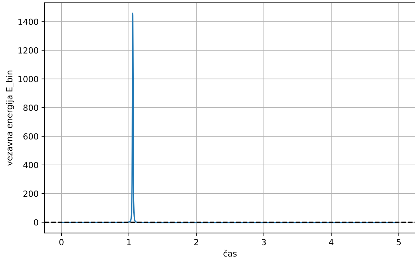
Vezavna energija dvozvezdja skozi čas ( a=0.5 , b=20 )
