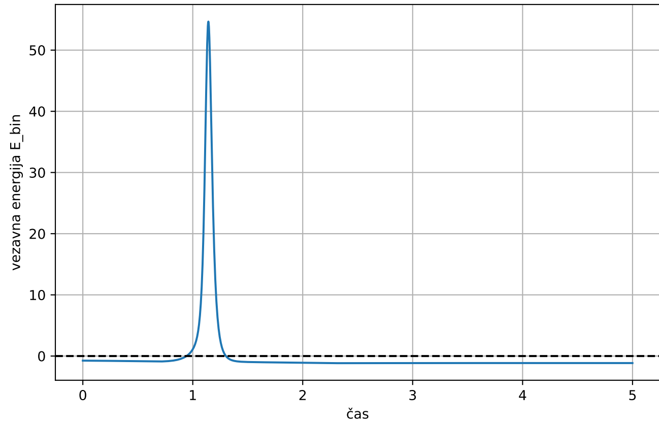
Vezavna energija dvozvezdja skozi čas ( a=1.0 , b=40 )
