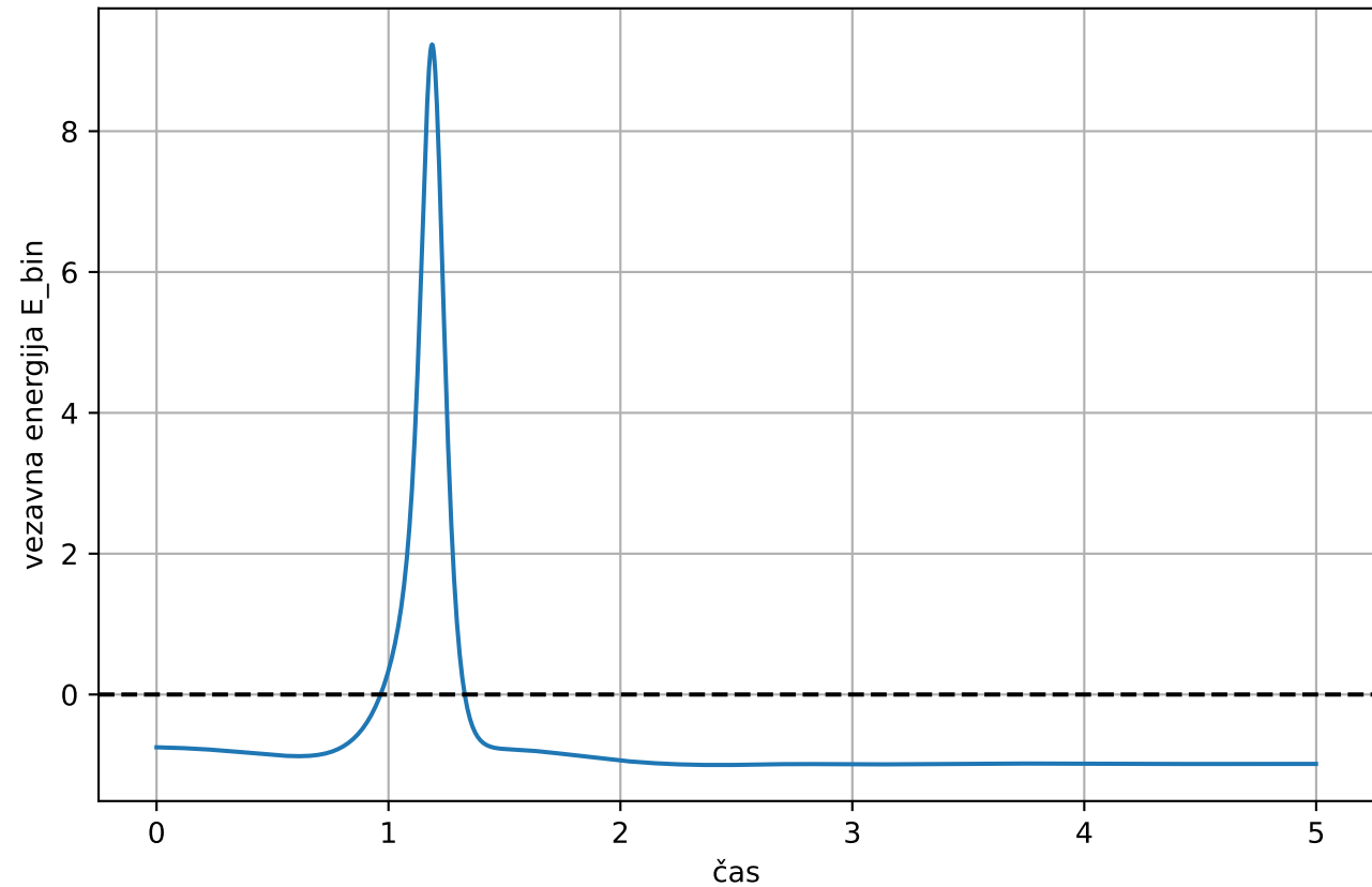
Vezavna energija dvozvezdja skozi čas ( a=1.0 , b=50 )
