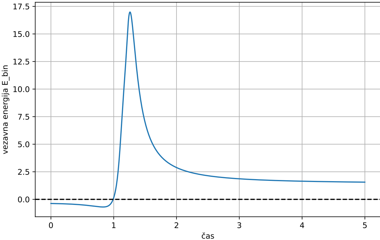
Vezavna energija dvozvezdja skozi čas ( a=2.0 , b=50 )
