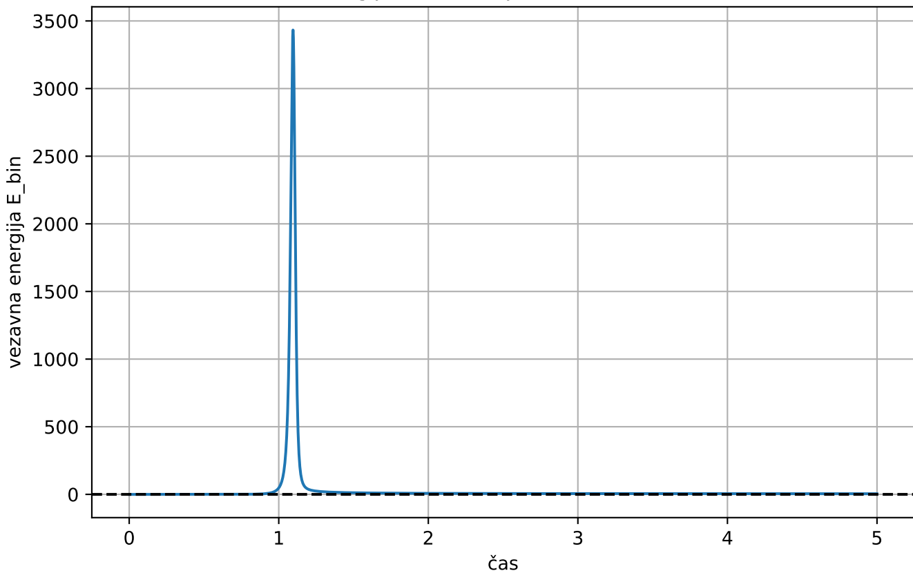
Vezavna energija dvozvezdja skozi čas ( a=3.0 , b=30 )
