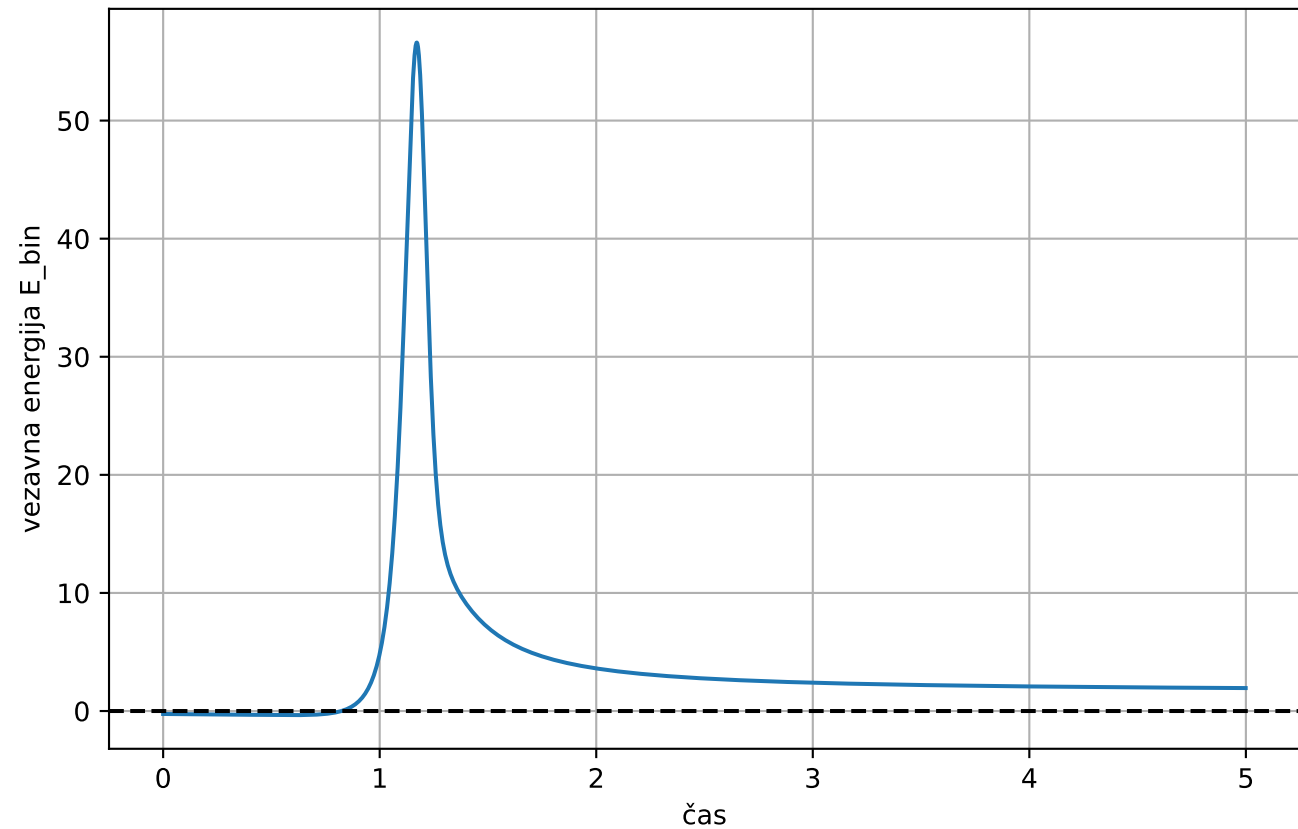
Vezavna energija dvozvezdja skozi čas ( a=3.0 , b=50 )
