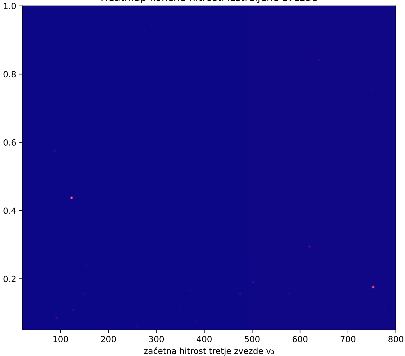
Heatmap končne hitrosti izstreljene zvezde
