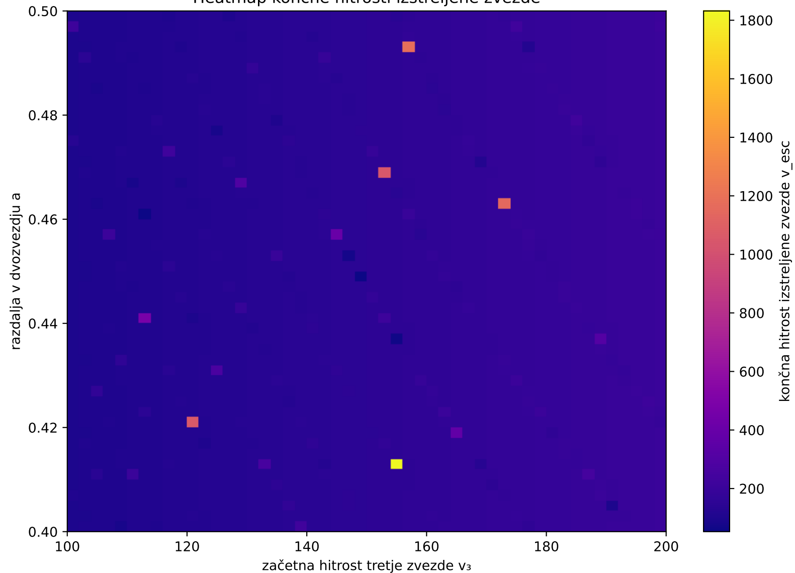
Heatmap končne hitrosti izstreljene zvezde
