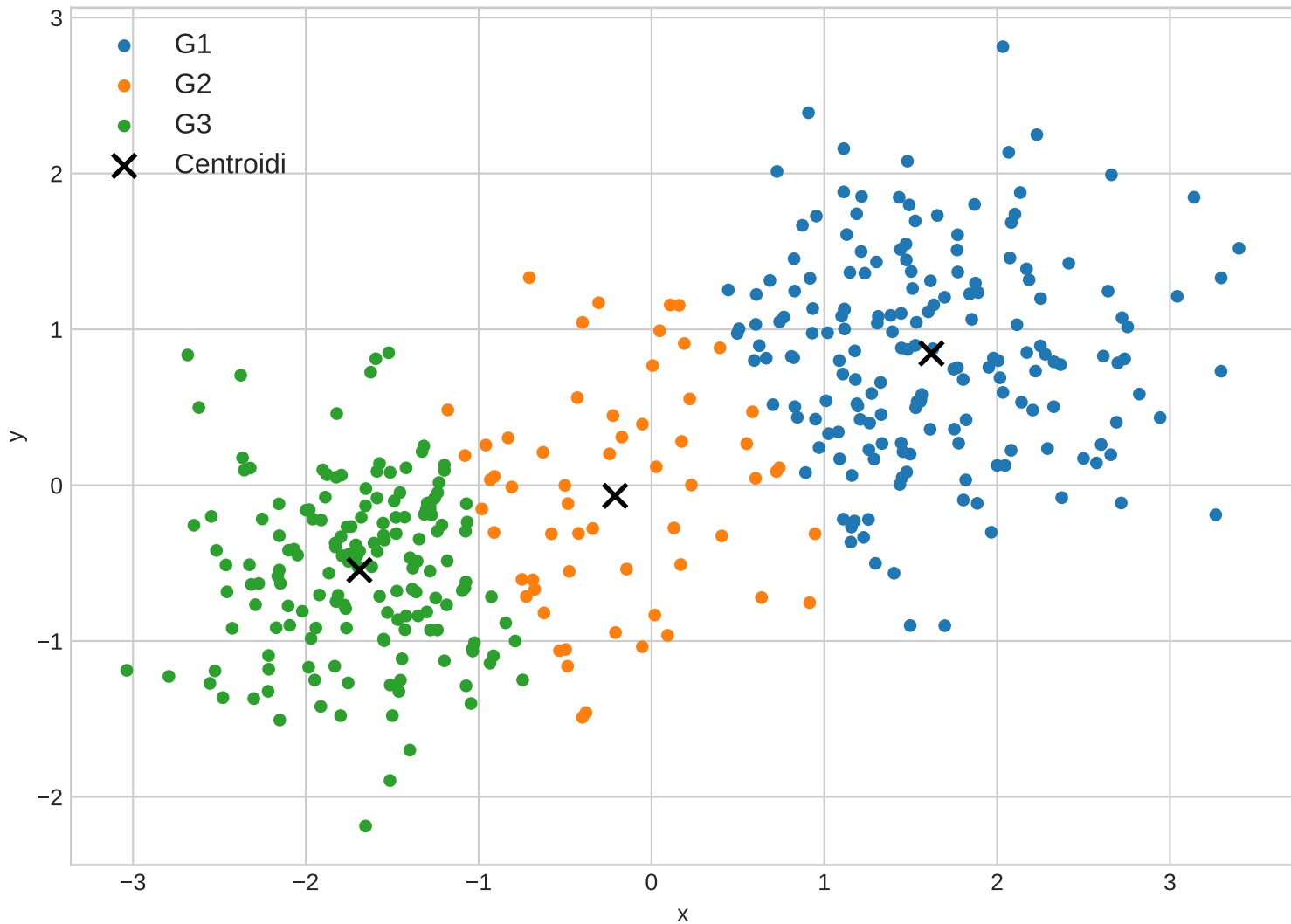
Lastna implementacija K-means (K = 3)
