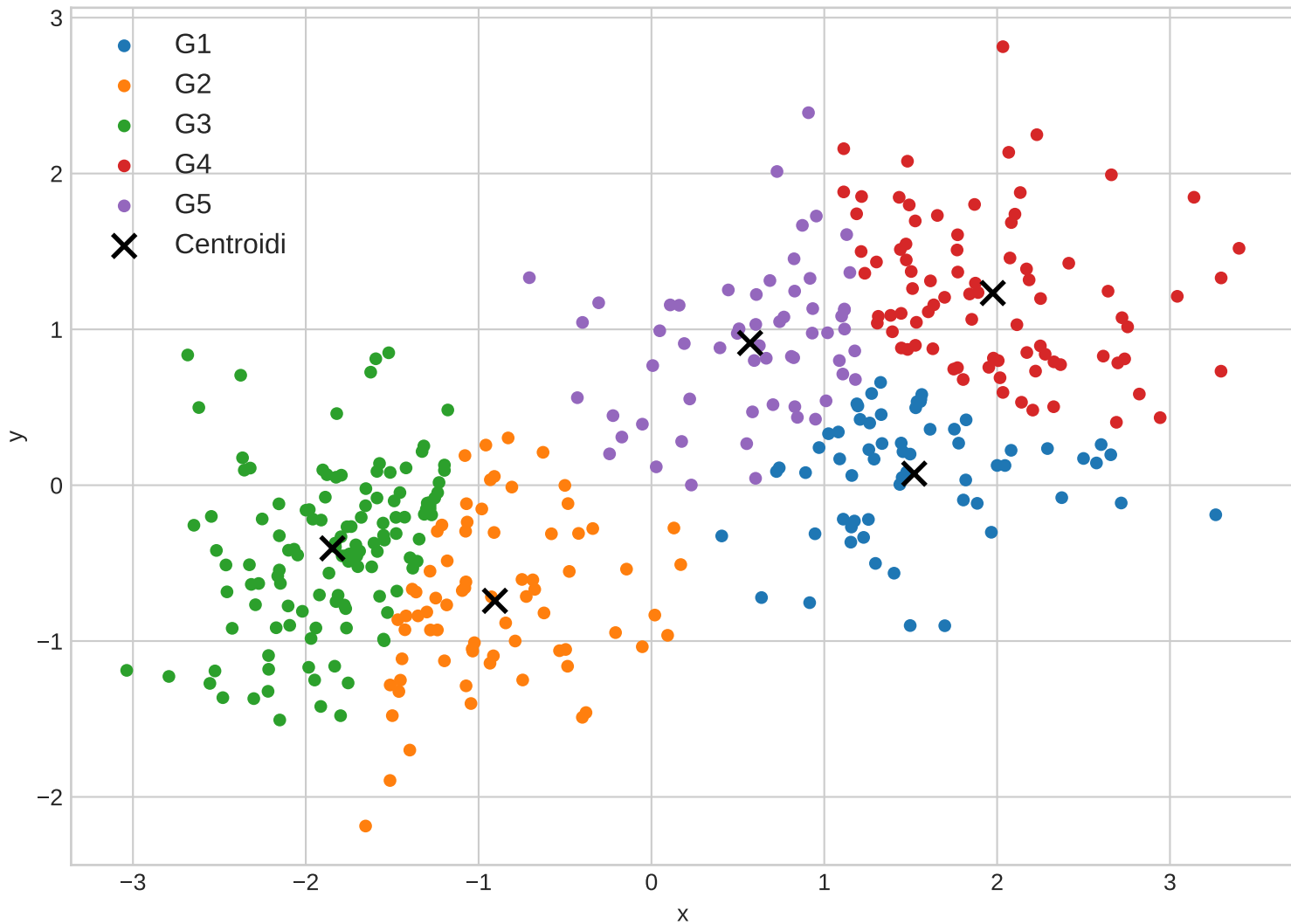
Lastna implementacija K-means (K = 5)
