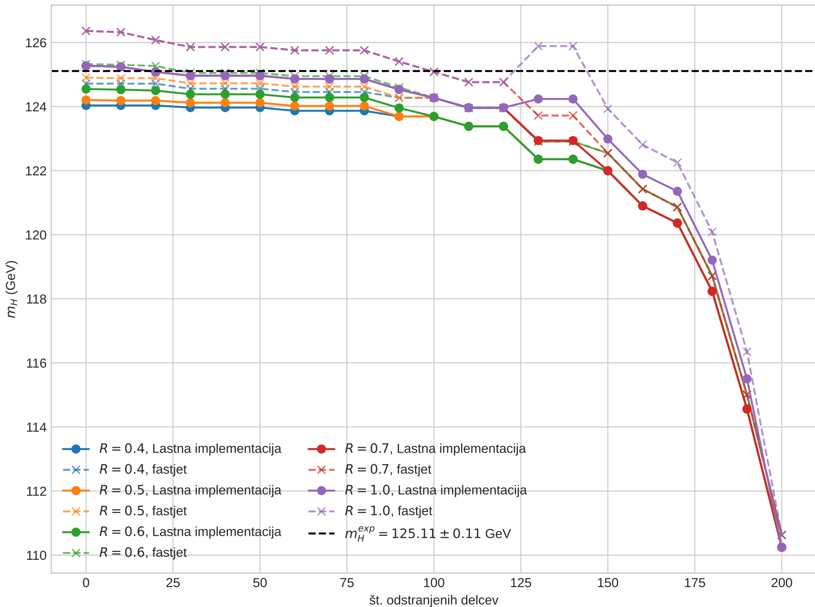
IR varnost: Lastna implementacija in fastjet k_t
