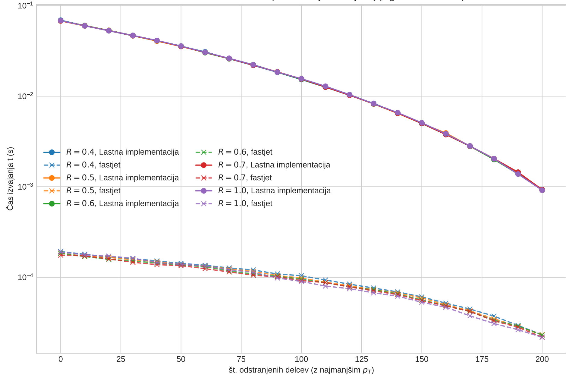
Časovna zahtevnost: Lastna implementacija in fastjet k_t (logaritemska skala)
