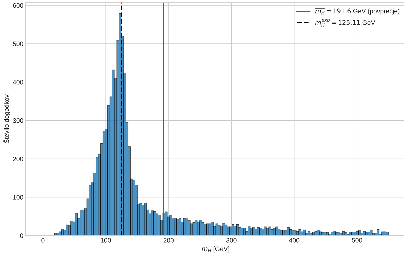
Histogram m_H iz algoritma fastjet k_t , R = 0.6
