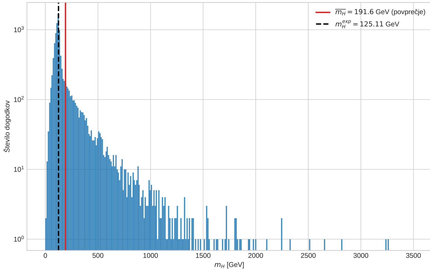
Histogram m_H iz algoritma fastjet k_t , R = 0.6 (logaritemska skala)
