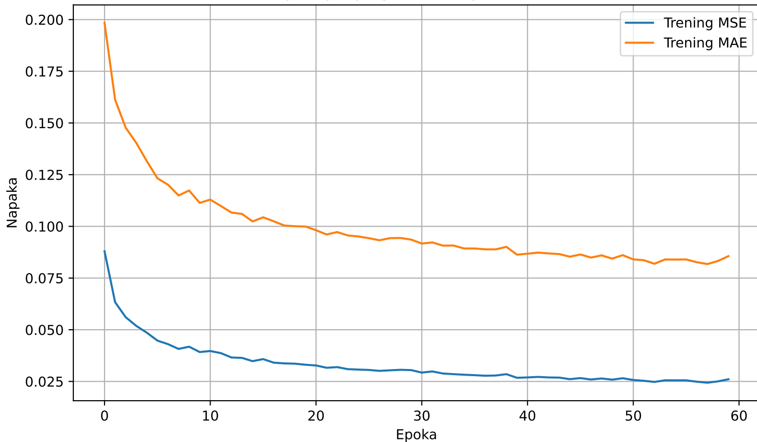
Učenje najboljšega modela po GridSearch
