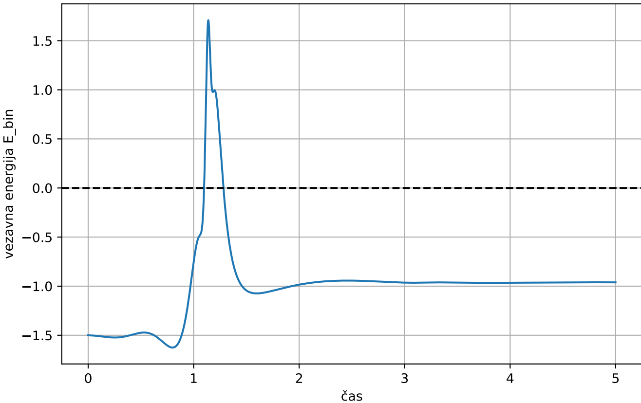
Vezavna energija dvozvezdja skozi čas ( a=0.5 , b=40 )
