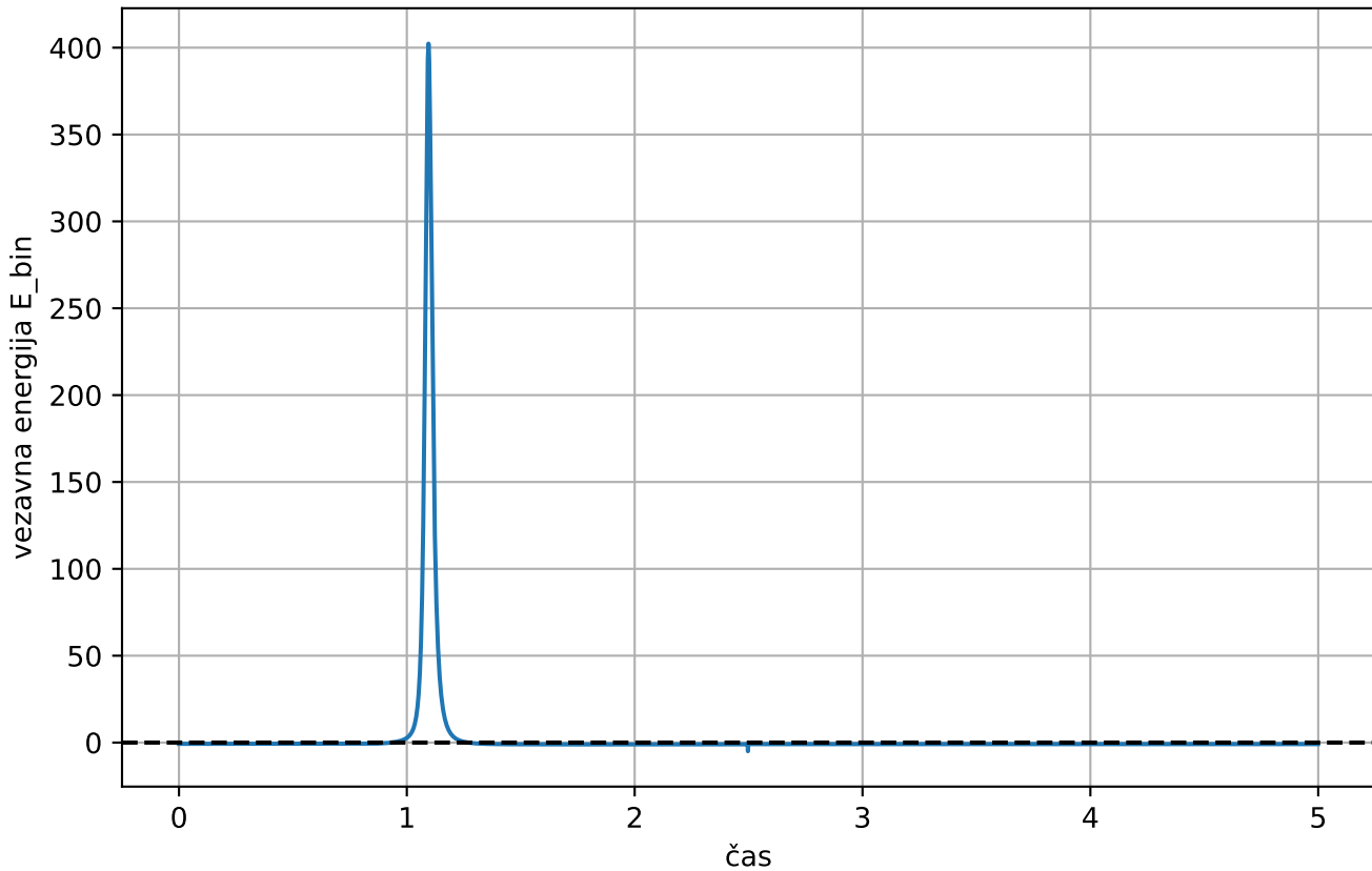
Vezavna energija dvozvezdja skozi čas ( a=1.0 , b=30 )
