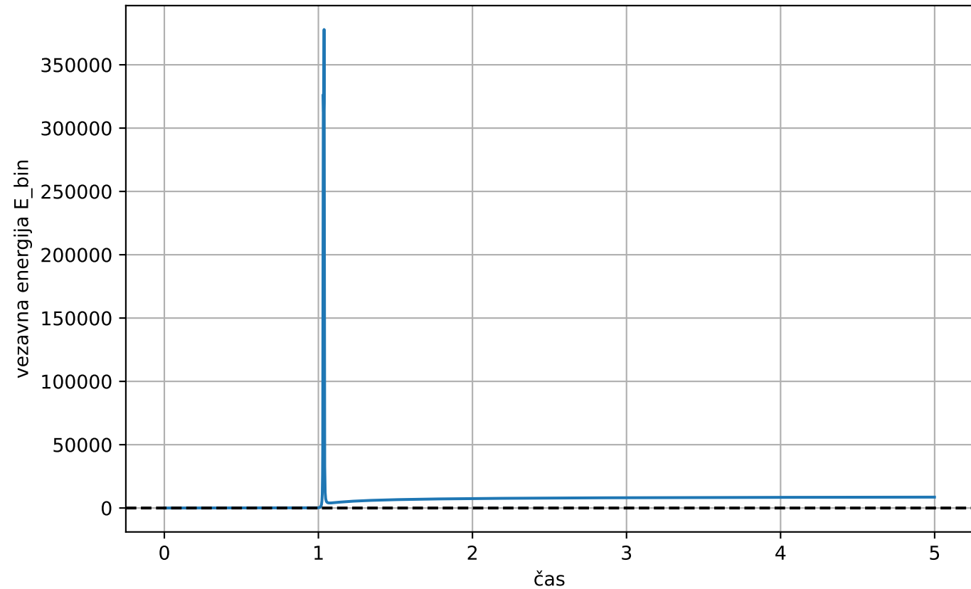
Vezavna energija dvozvezdja skozi čas ( a=2.0 , b=10 )
